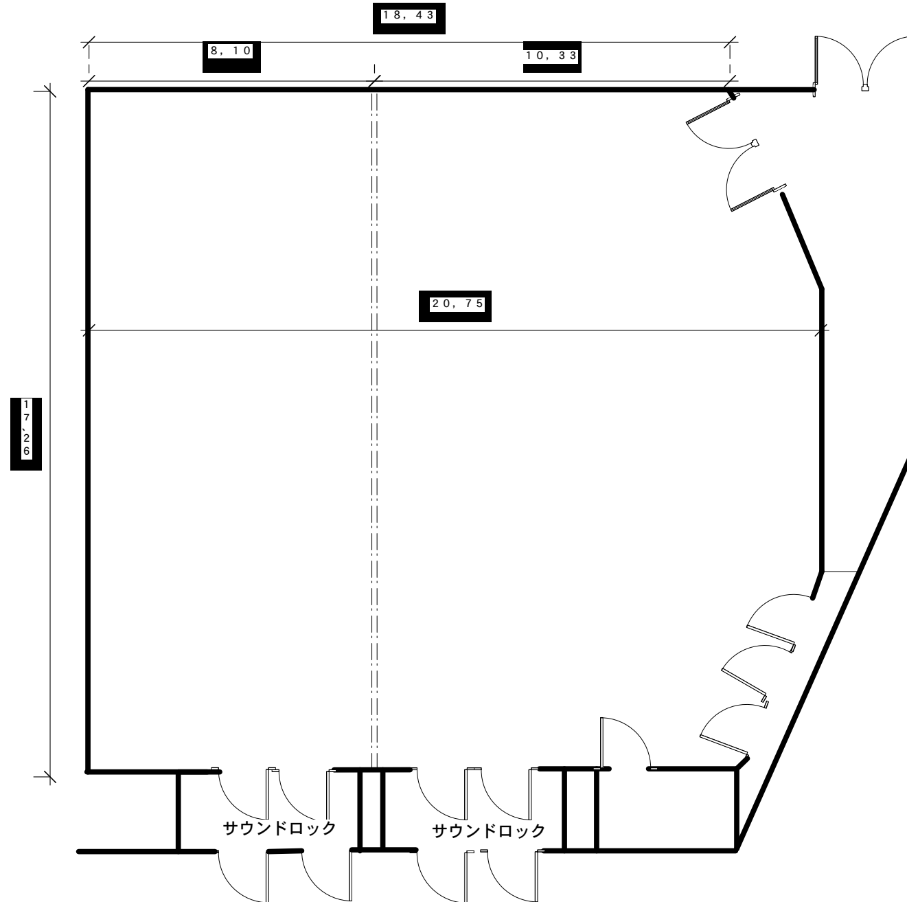
須崎市立市民文化会館大会議室兼展示ホール平面図 s = 1/100
